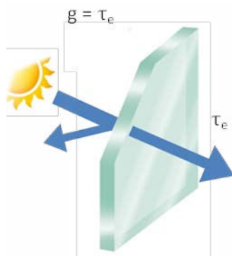
FIGURA 12. SCHEMA DI TRASMISSIONE SOLARE ATTRAVERSO UNA VETRATURA ISOLANTE
