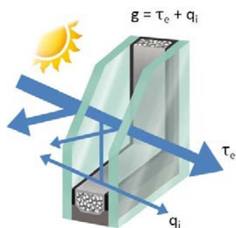
FIGURA 12. SCHEMA DI TRASMISSIONE SOLARE ATTRAVERSO UNA VETRATURA ISOLANTE
